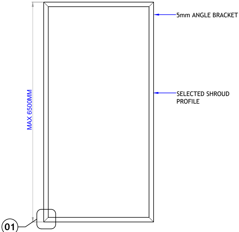
ELEVATION
