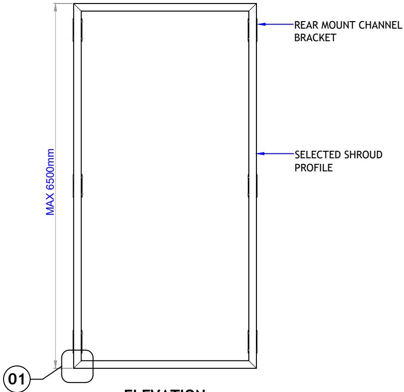
ELEVATION
